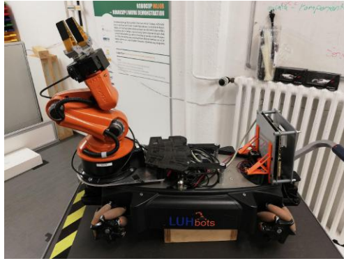
(a) LUHbots youBot
