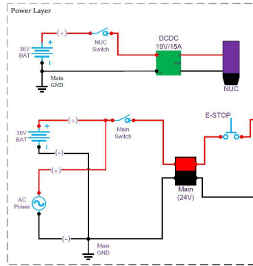
Fig. 2. Power Layer
