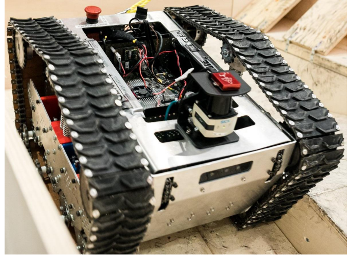
Fig. 1. Photo our robot at the 2019 open house of École de Technologie Supérieure
