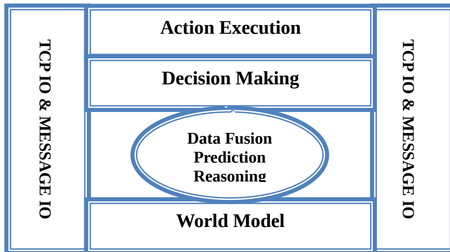
Fig.1. Code structure of SEU_RedSun
