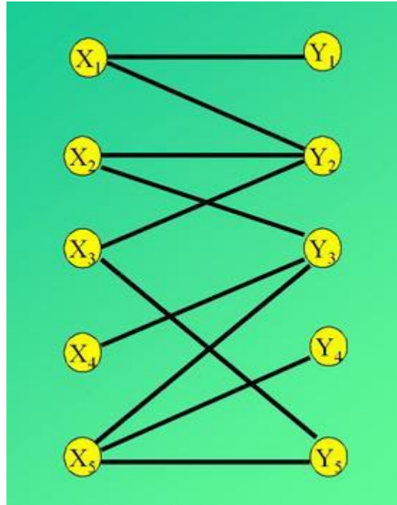
Fig.6 bipartite graphs
