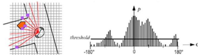
Fig. 3. VFH output [6]
