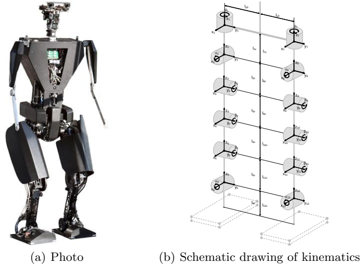
Fig. 1. Humanoid robot TULip
