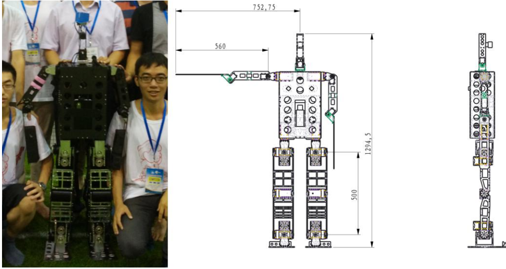
Fig. 1. 1) Strider Pro robots 2) Robot Dimension
