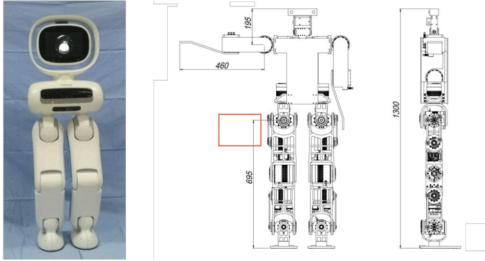
Fig. 1. 1) Walker robot 2) Robot Dimension
