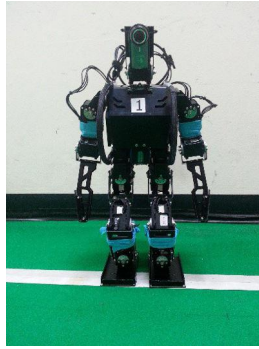
Fig.1. 'Hanuman' striker robot.
