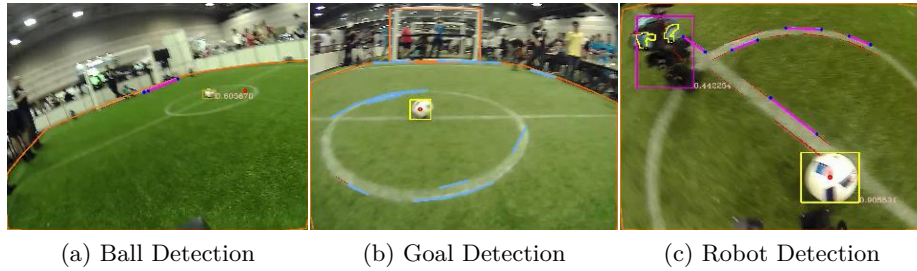
Fig. 5: Obejt detection
