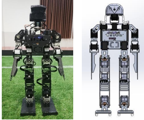
Fig. 1. Ashkan humanoid KidSize robot.
