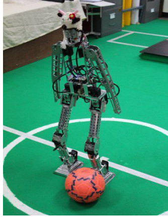
Fig. 1. Ka-Ti (Goalie)
