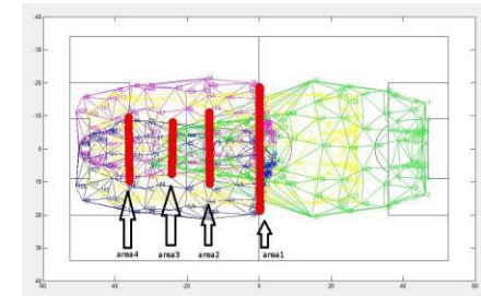
Fig 6 Gliders2014 2,3,6,11 formation
