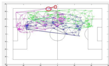
Fig 7 Helios2014 4,7,9 formation
