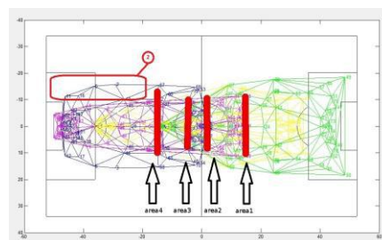
Fig 8 Helios2014 2,3,6,11 formation
