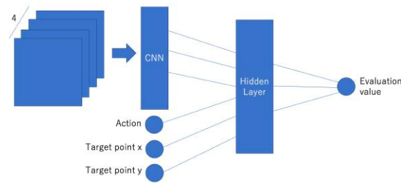
Fig. 2. CNN model
