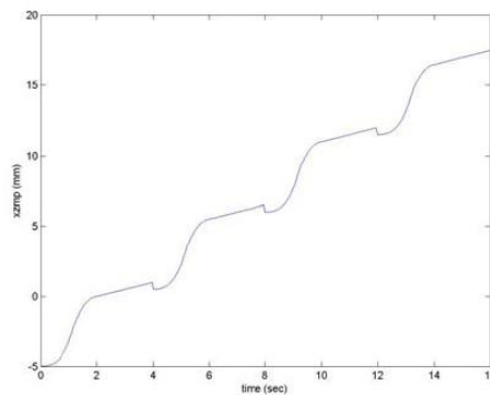
Fig.6 ZMP trajectory
